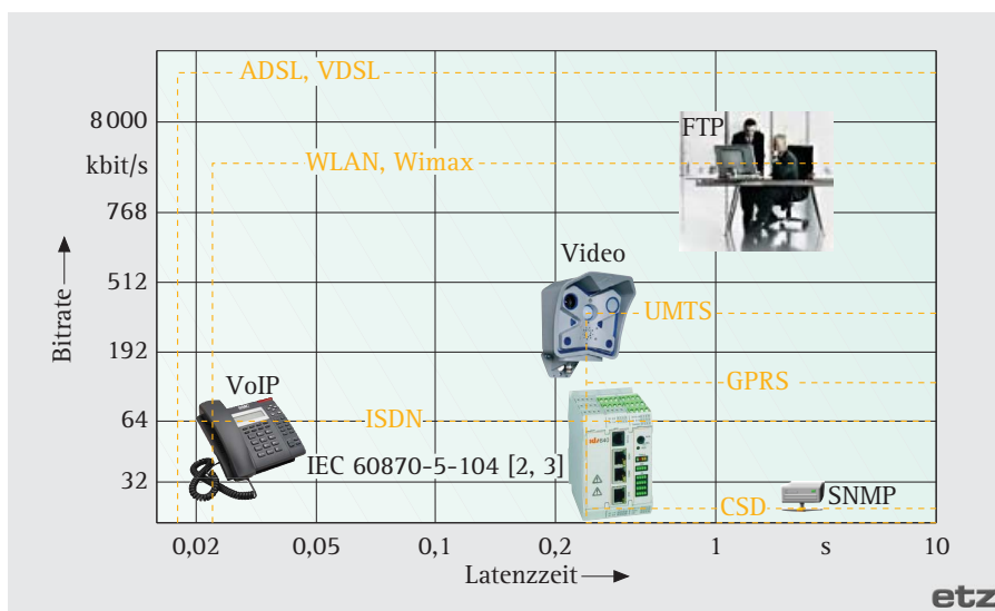
Bild 2. Vergleich der Dienstgüte (QoS) unterschiedlicher Übertragungsdienste
