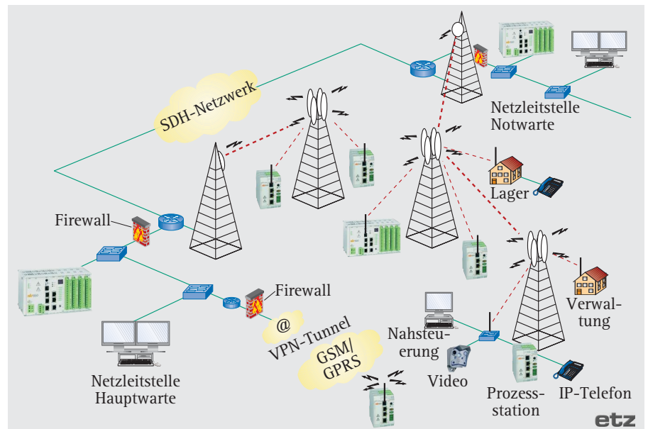
Bild 1. Typische Struktur von WLAN- und Wimax-Netzen
