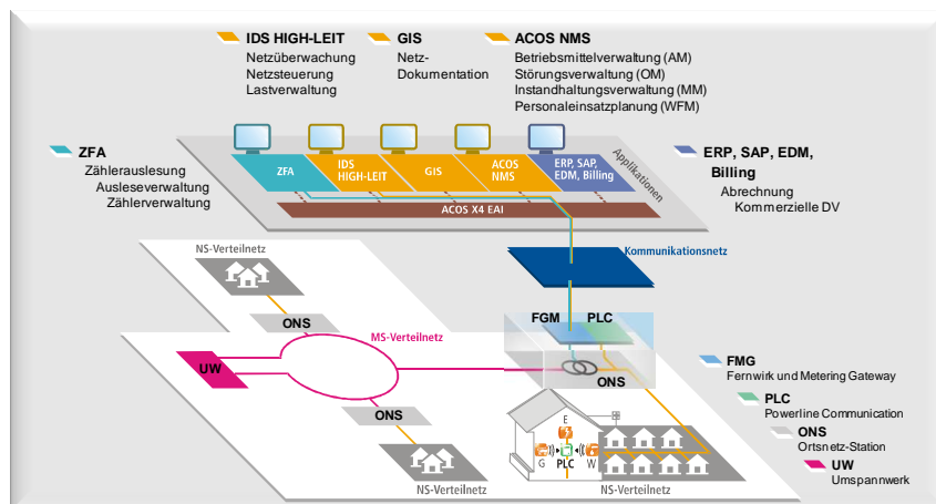
Darstellung: Systemübersicht SMART - Grid - Metering - Home mit ACOS NMS & ACOS X4
