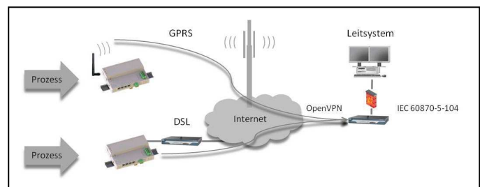
Darstellung: ACOS 710 / 720 über DSL und GPRS
