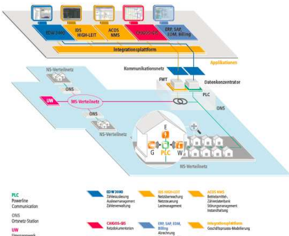
Abbildung: Systemkonzept Smart-Grid-Metering
