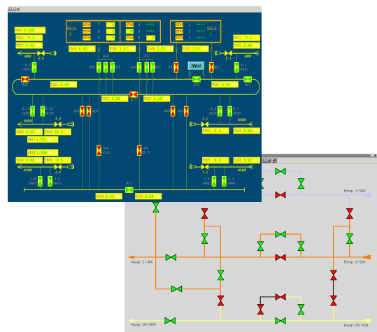
Abbildungen: Webinterface & Rohrnetztopologie
